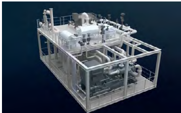
LNG추진선 연료공급시스템
